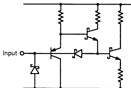
Fig. 3 – MB7117/7118 INPUT
