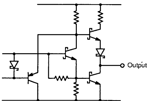
Fig. 5 – MB7118 OUTPUT
