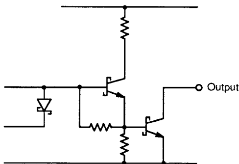
Fig. 4 – MB7117 OUTPUT
