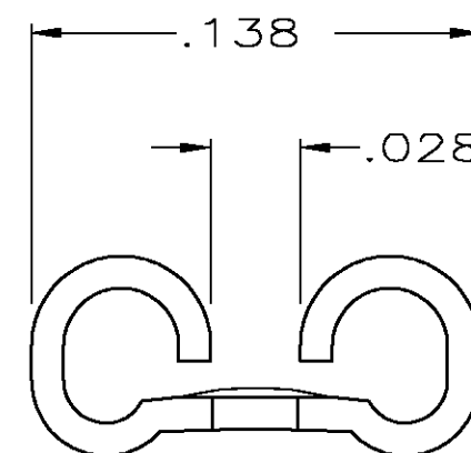
VIEW A-A
