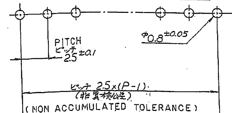
基板加工寸法 FIG.2
