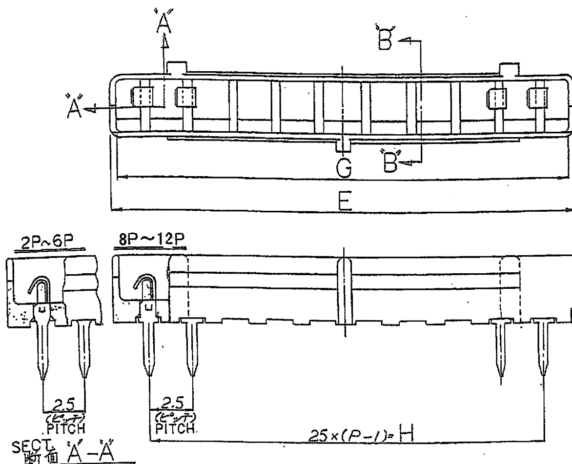
P.C.B. LAYOUT FIG.2
