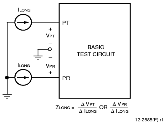
Figure 9. Longitudinal Impedance
