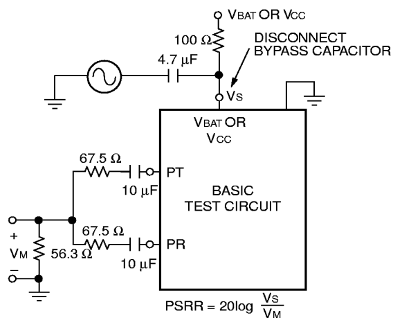
Figure 7. Longitudinal PSRR
