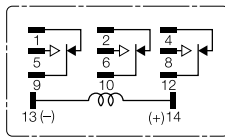
3PDT
